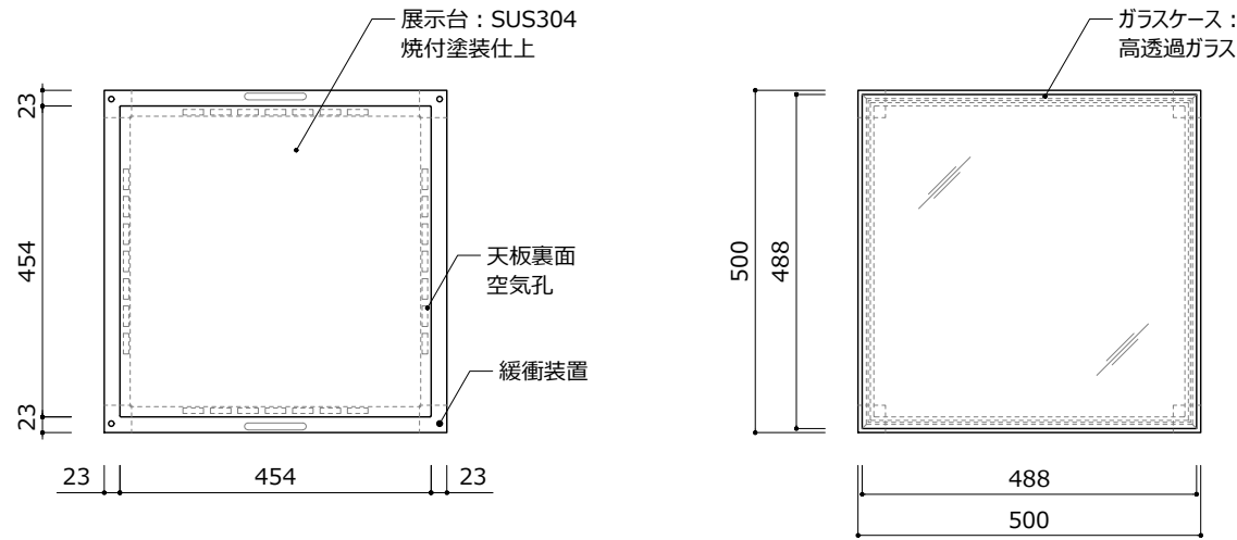
平面
