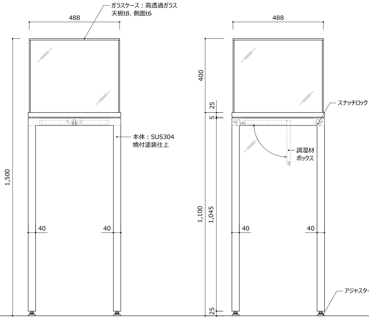
側面
