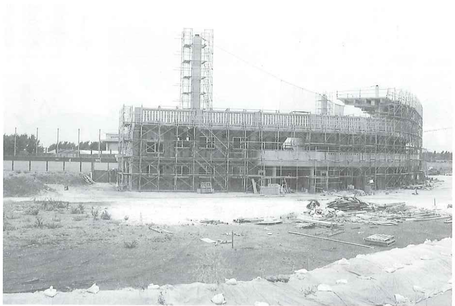
建設中の久米島野球場
